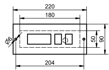
Steuerungspanel Panneau de commande Control panel
